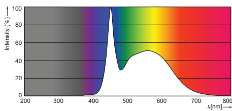
LEDtube 600mm 8W /865, 1200mm 16W /865
