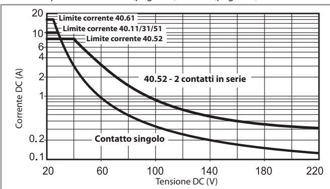
H 40.2 - Massimo potere di rottura su carichi in DC1
