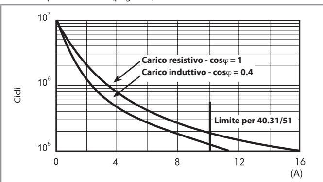
F 40.5 - Durata elettrica (AC) in funzione della corrente
