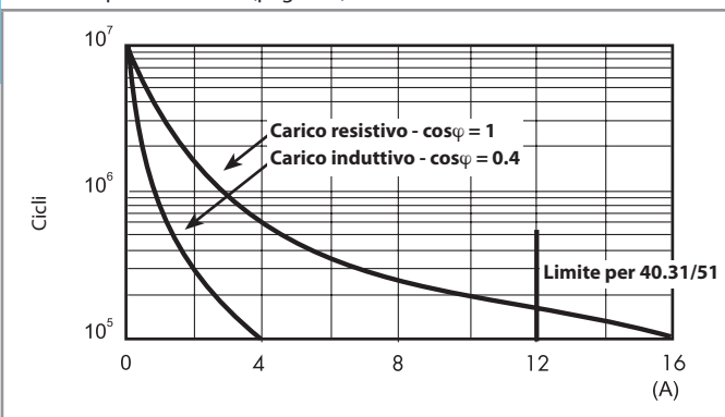
F 40.3 - Durata elettrica (AC) in funzione della corrente
