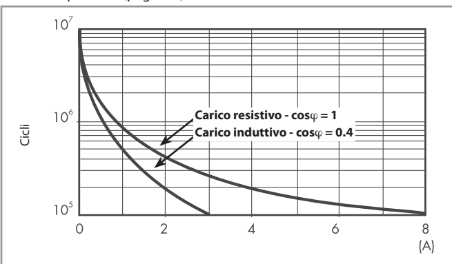
F 40.4 - Durata elettrica (AC) in funzione della corrente
