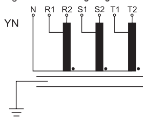
Schema dell'avvolgimento - Winding diagram
