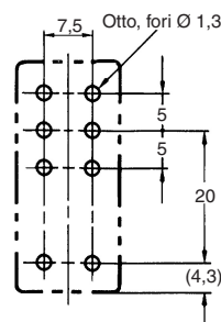
Fori di montaggio
