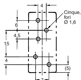
Disposizione terminali (vista dal basso)
