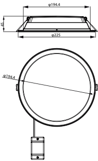
DN065B G4 LED20/830 19W 220-240V D200 RD
