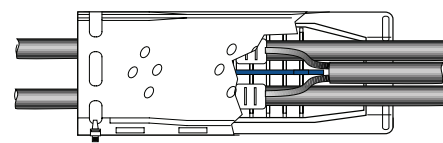
Giunzione in derivazione tra due cavi unipolari ed un cavo bipolare
